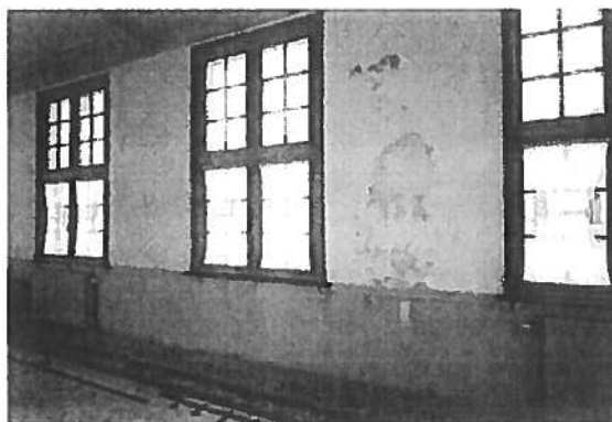
vochtdoorslag wanden Eerste Kamer
