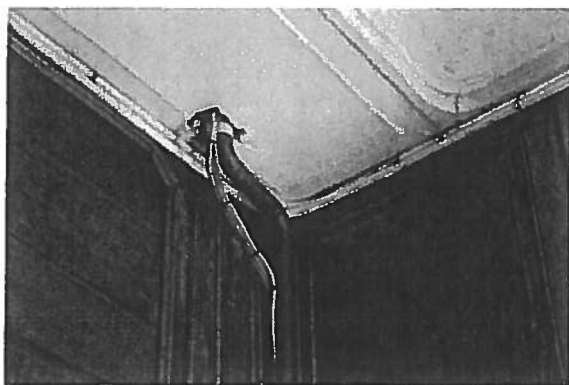
alternatieve kabel- en leidingtracé als gevolg van slechte bereikbaarheid installaties ambtenarenkamer Eerste Kamer
