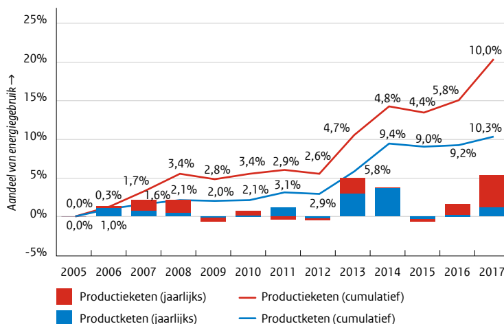
Figuur 3.7 – Besparing door ketenefficiëntie MJA3-convenant vanaf 2005
