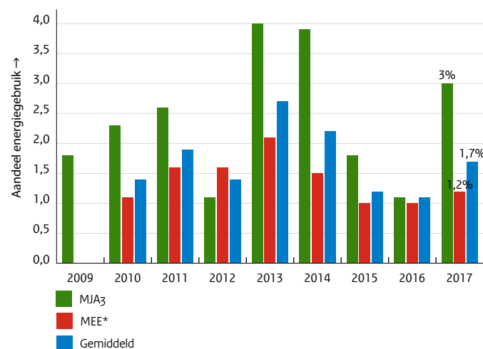
Figuur 1.1 – Jaarlijkse verbetering in landelijk resultaat in % van het eigen energiegebruik
