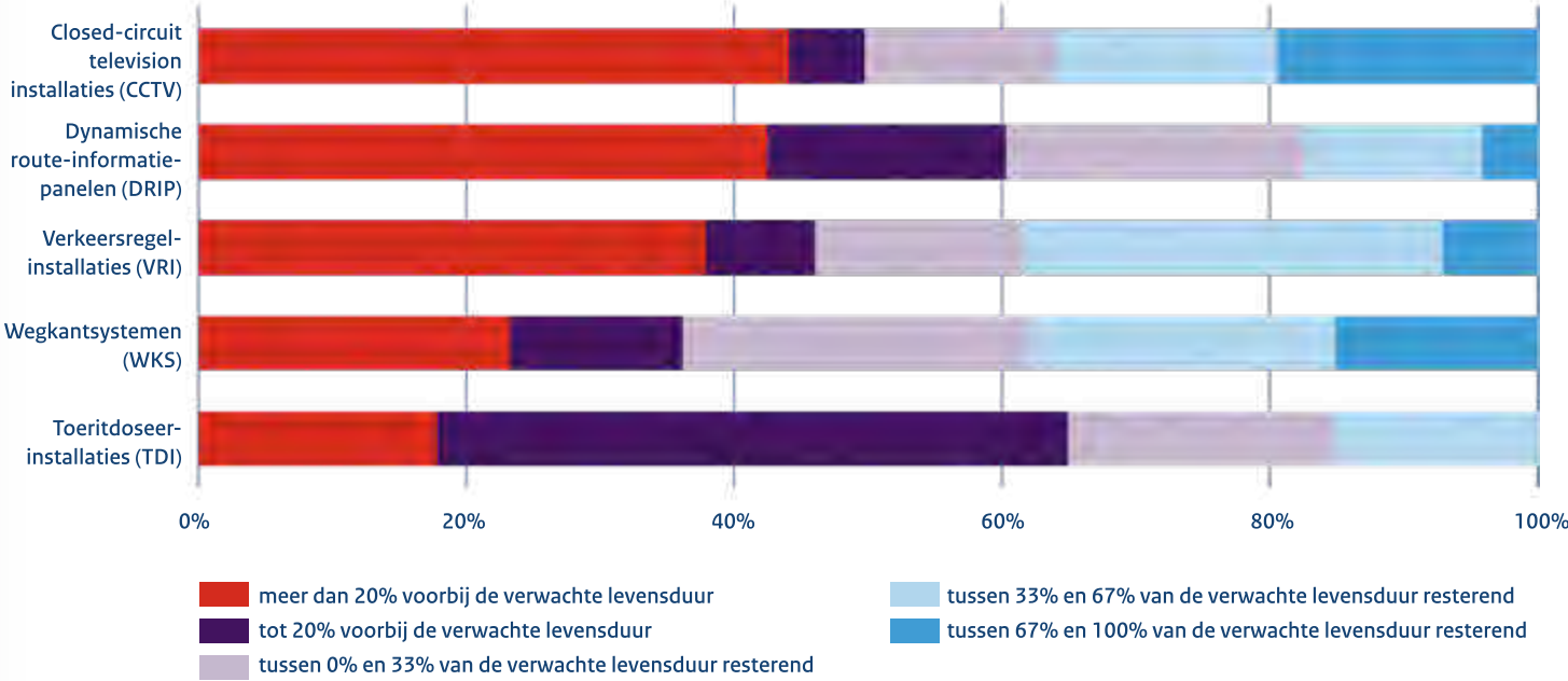
Figuur 10: Verwachte resterende levensduur Dynamisch Verkeersmanagement HWN gewogen naar vervangingswaarde (peildatum: 1 januari 2026)
