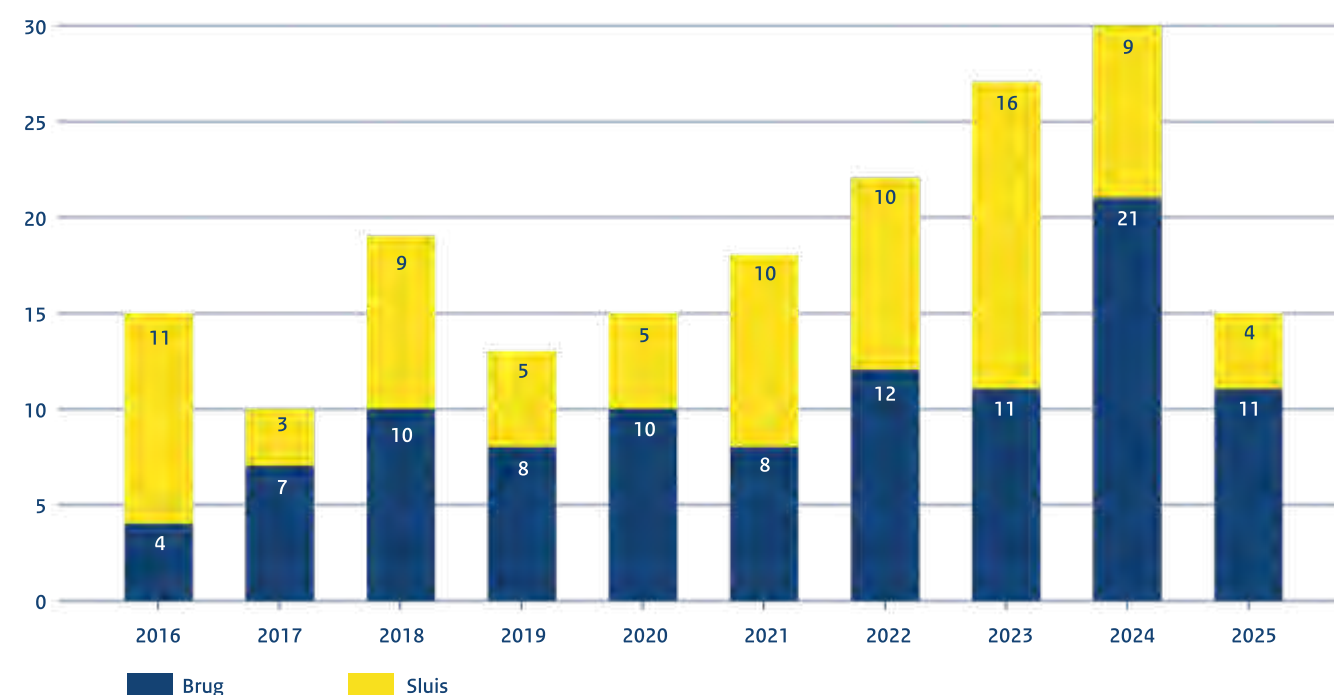
Figuur 20: Significante scheepsongevallen bij bruggen en sluizen op het RWS-areaal
