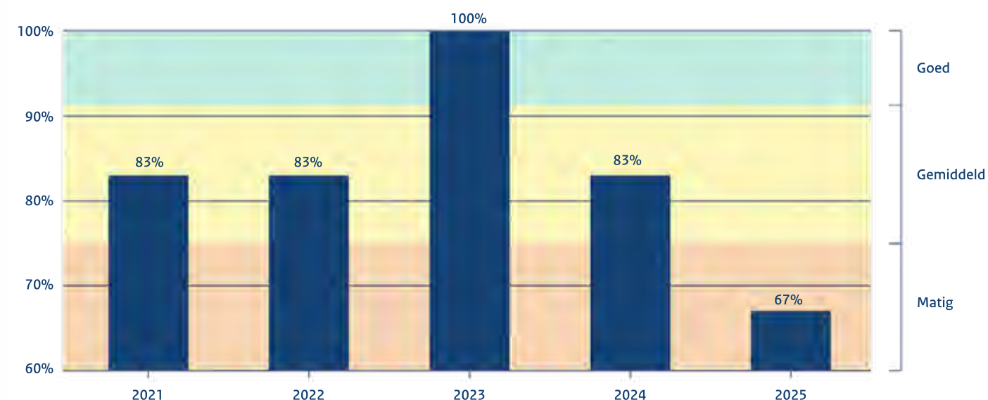
Figuur 26: De ontwikkeling van de veiligheid van de stormvloedkeringen van het HWS van 2021 t/m 2025
