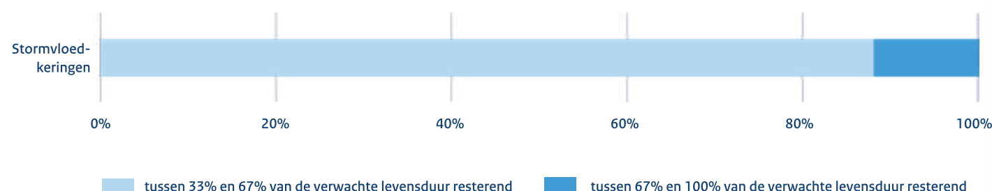
Figuur 28: Verwachte resterende levensduur stormvloedkeringen gewogen naar vervangingswaarde (peildatum: 1 januari 2026).
