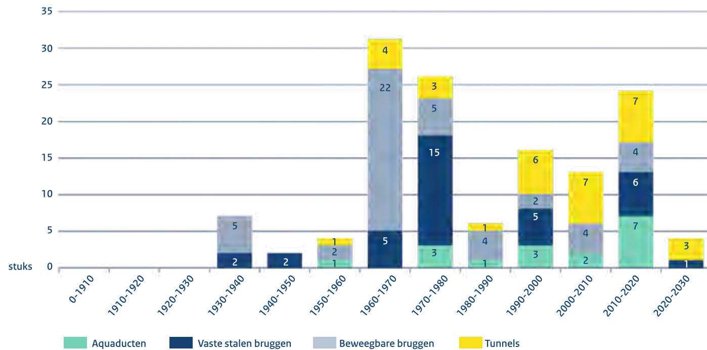
Figuur 2: Jaren van aanleg kunstwerken HWN: tunnels, beweegbare bruggen, vaste stalen bruggen en aquaducten (peildatum: 1 januari 2026)
