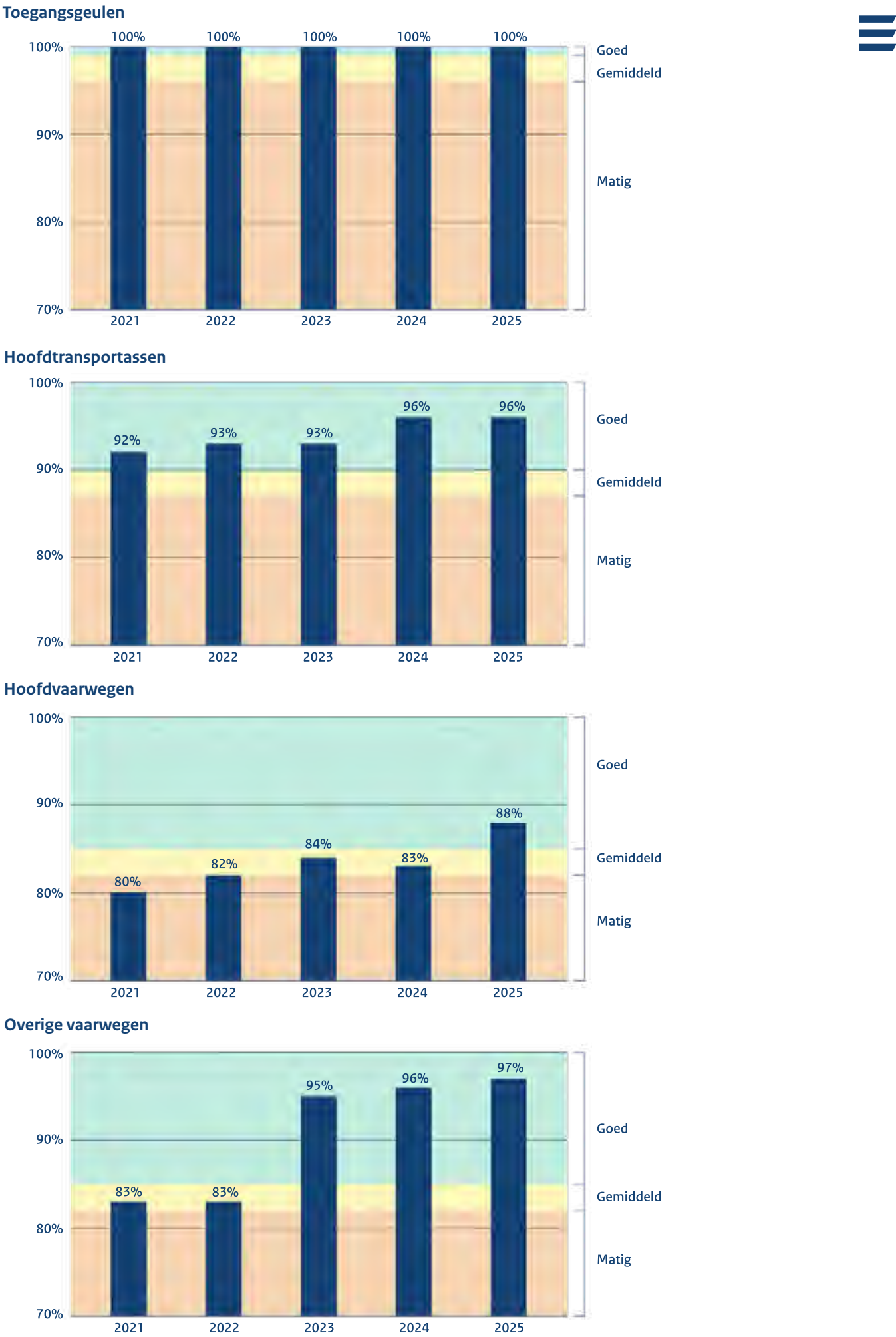
Figuur 19: De ontwikkeling van de technische conditie op de bodems van de vaargeulen van HVWN van 2021 t/m 2025
