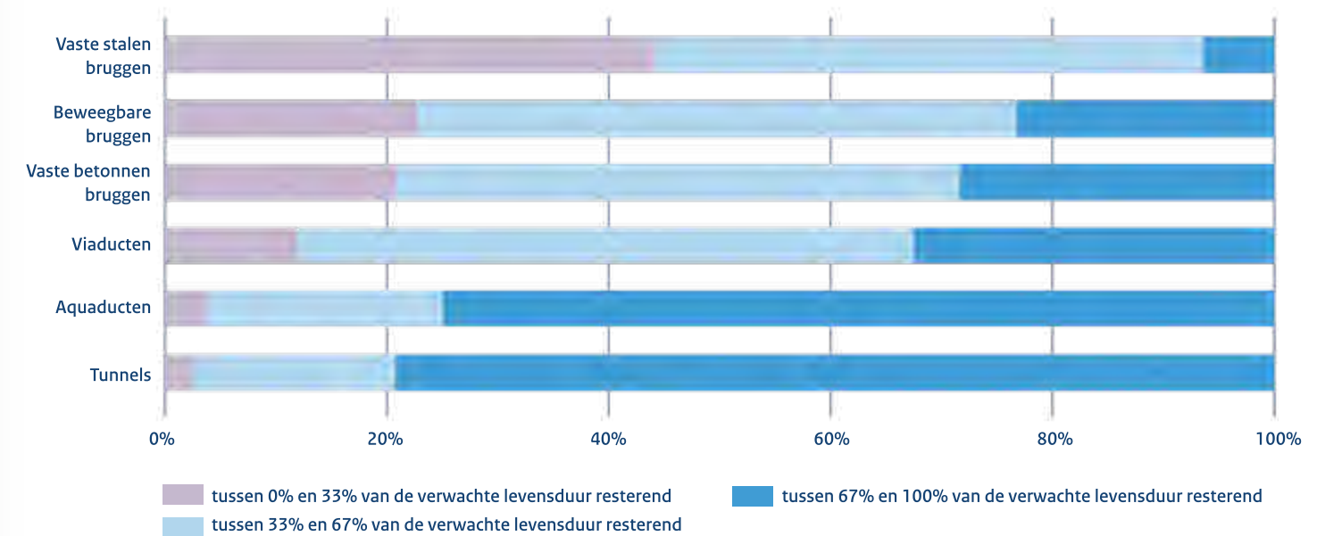
Figuur 4: Verwachte resterende levensduur kunstwerken gewogen naar vervangingswaarde HWN (peildatum: 1 januari 2026).
