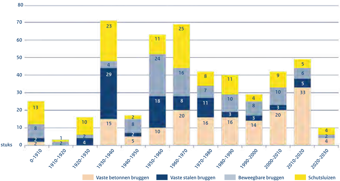
Figuur 13: Jaren van aanleg kunstwerken HVWN (peildatum: 1 januari 2026)
