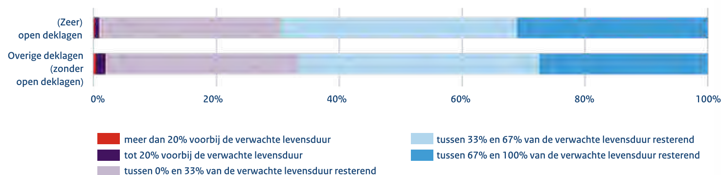
Figuur 7: Verwachte resterende levensduur verhardingen HWN gewogen naar vervangingswaarde (peildatum: 1 januari 2026)
