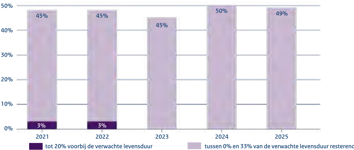
Figuur 21: De ontwikkeling van de verwachte resterende levensduur op de kunstwerken van het HWS van 2021 t/m 2025
