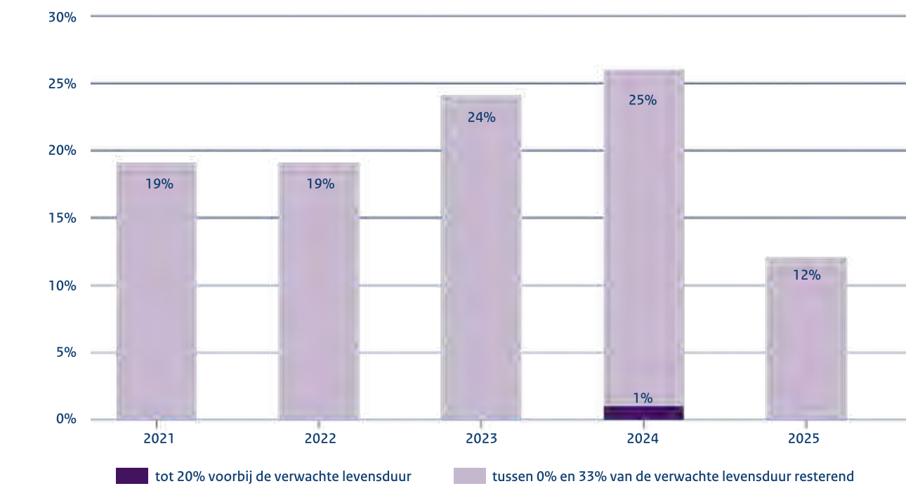
Figuur 1: De ontwikkeling van de verwachte resterende levensduur op de kunstwerken van het HWN van 2021 t/m 2025
