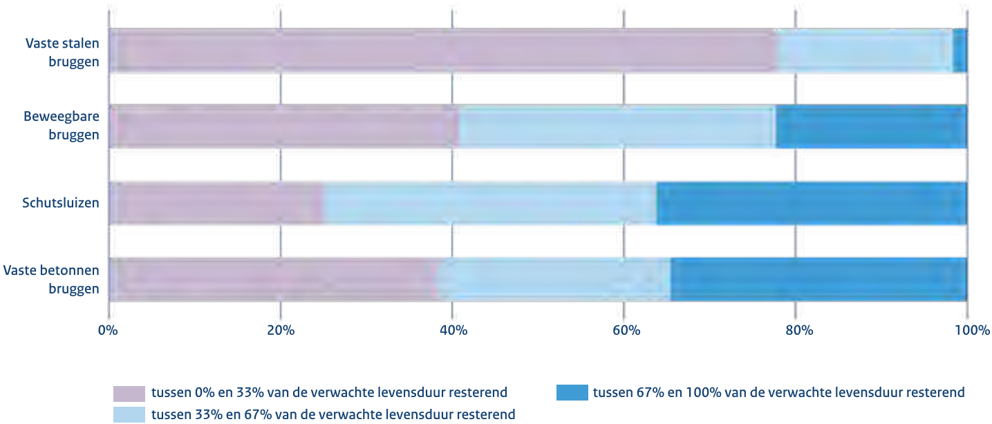
Figuur 14: Verwachte resterende levensduur kunstwerken gewogen naar vervangingswaarde HVWN (peildatum: 1 januari 2026)
