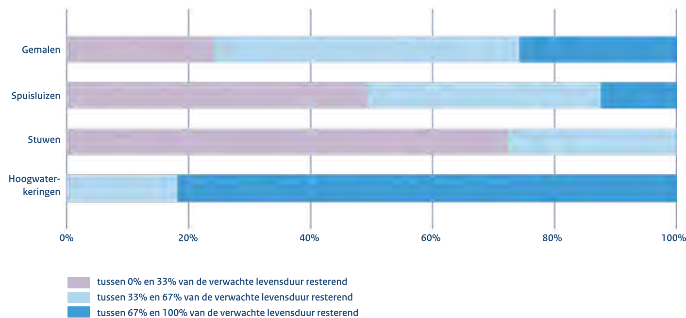
Figuur 23: Verwachte resterende levensduur kunstwerken HWS gewogen naar Vervangingswaarde (peildatum: 1 januari 2026)
