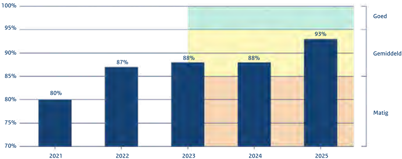
Figuur 29: De ontwikkeling van de veiligheid op de uiterwaarden van HWS van 2021 t/m 2025
