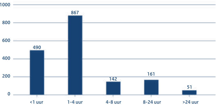
Figuur 16: Storingsduur in het jaar 2025. Op de x-as staat de storingsduur in klassen, op de y-as hoe vaak deze duur is voorgekomen
