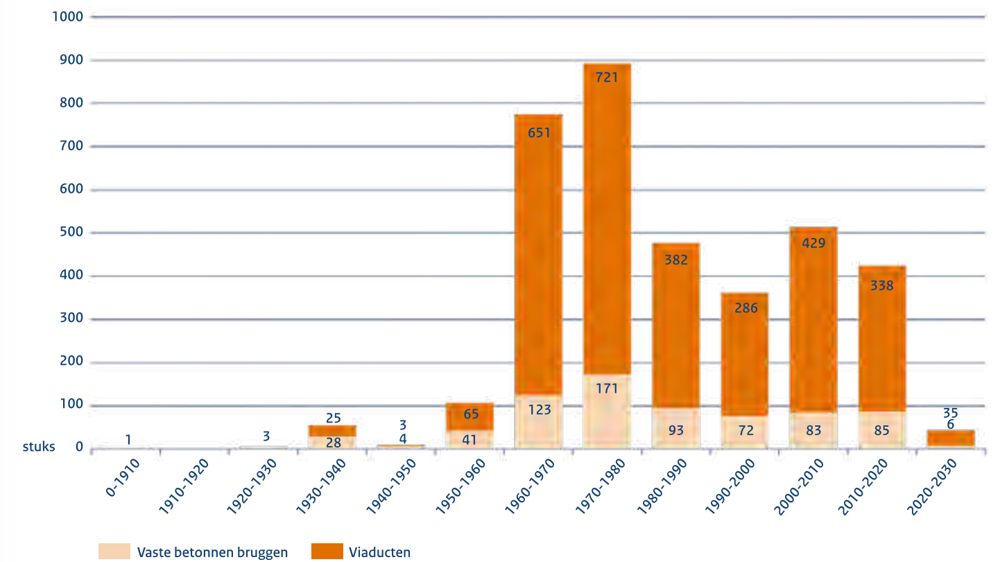
Figuur 3: Jaren van aanleg kunstwerken HWN: viaducten en vaste betonnen bruggen (peildatum: 1 januari 2026)
