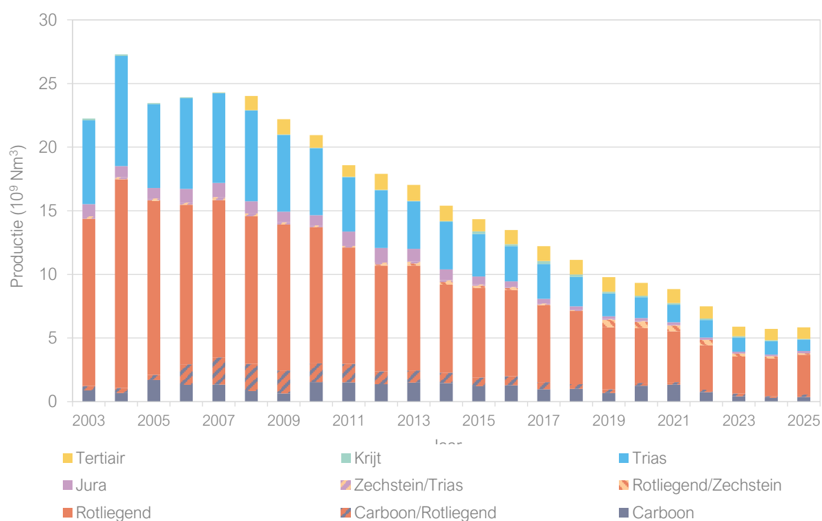
Figuur 3.3 Gasproductie op zee, per reservoir.
