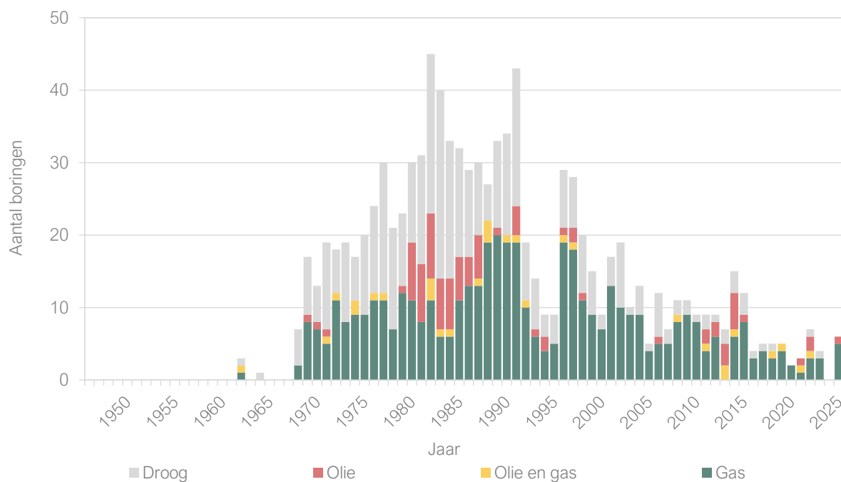
Figuur 11.2 Verloop van exploratie- en evaluatieboringen voor koolwaterstoffen op zee vanaf 1946.
