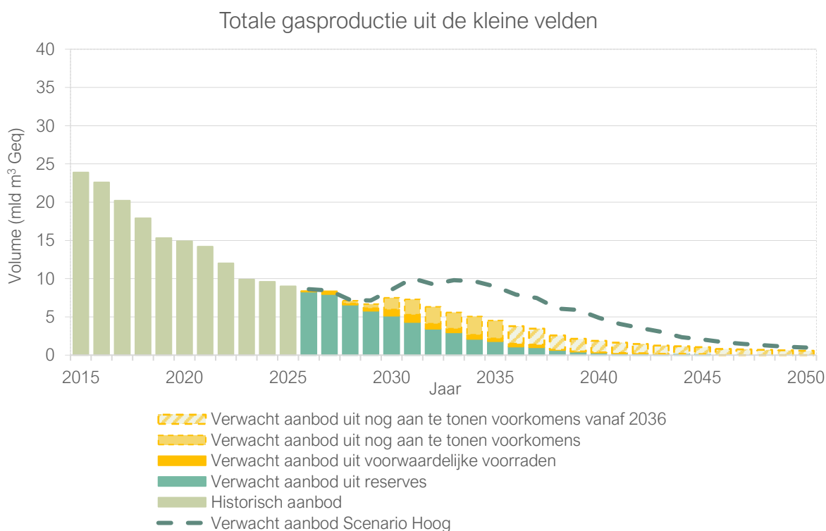
Figuur 1.7 Totale gaswinning uit de kleine velden. Gerealiseerde (2015-2025) en verwachte (2026 – 2050) winning van aardgas uit de kleine velden voor zowel land als zee. De voorraden worden conform het Midden scenario gepresenteerd. Het kussengas van gasopslagen is hier buiten beschouwing gelaten. De cumulatieve prognose voor het Hoog scenario wordt weergegeven als groene stippellijn. De waarden onderliggend aan dit profiel worden in Excel overzicht tabbladen B, C en F gegeven.
