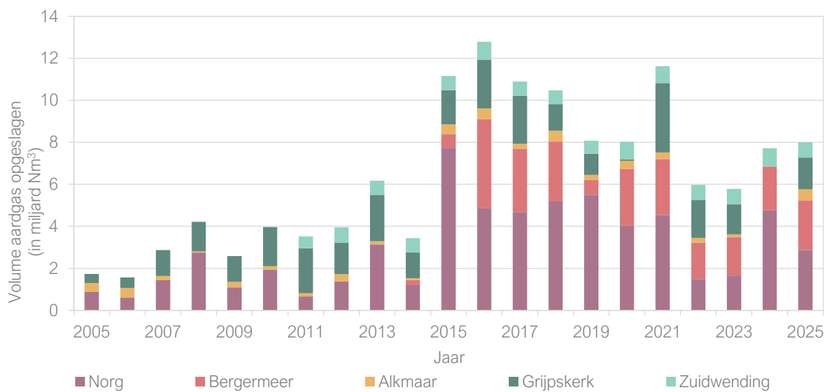
Figuur 4.1 Opgeslagen volume aardgas per UGS-locatie van 2005-2025.
