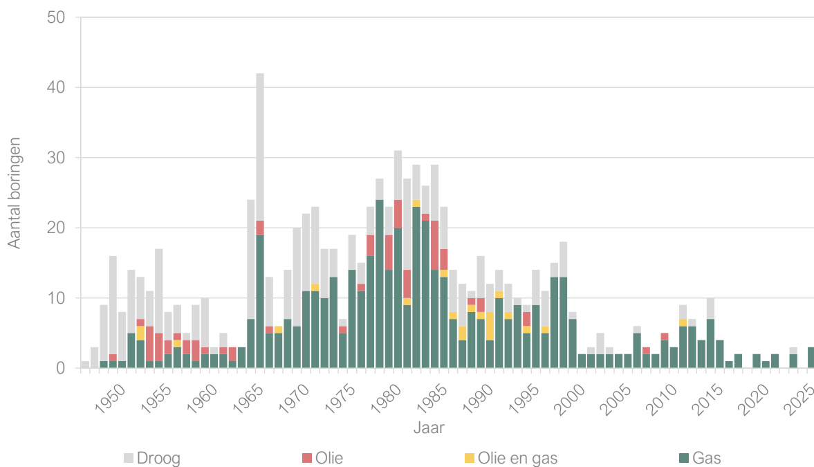
Figuur 11.1 Verloop van exploratie- en evaluatieboringen voor koolwaterstoffen op land vanaf 1946.
