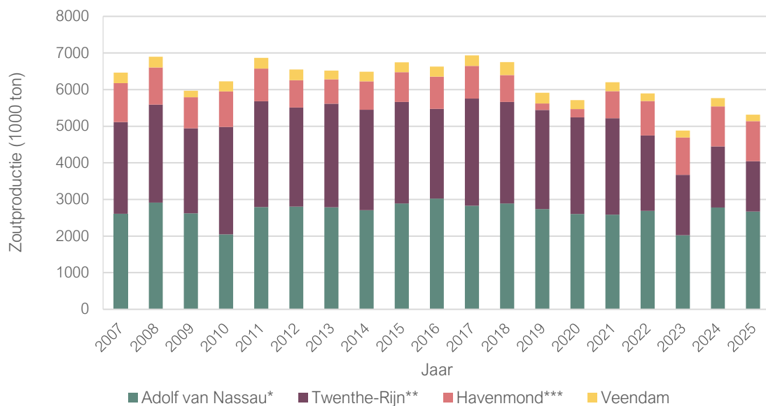
Figuur 6.1 Zoutproductie 2007 – 2025 (in 1000 ton), de productiegegevens zijn gebaseerd op cijfers die door de operators zijn verstrekt.
