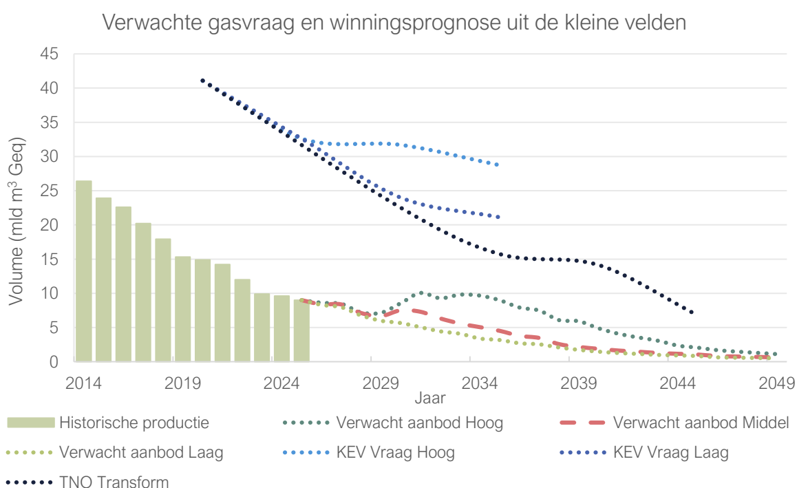
Figuur 1.8 De Nederlandse gasvraagontwikkeling en gaswinningprognoses voor de komende 25 jaar. De gasvraagontwikkeling is conform de geformuleerde beleidskeuzes opgesteld (KEV 2024). De KEV Vraag Hoog betreft de bovenkant van de bandbreedte van de raming op basis van alleen het vastgesteld en voorgenomen beleid, de KEV Vraag Laag de onderkant van de bandbreedte van dezelfde raming. Het TNO TRANSFORM scenario is ter aanvulling opgenomen omdat dit voldoet aan de broeikasgasneutraliteit in 2050 doelstelling. Voor de conversie van volume naar energie-eenheid is 1 miljard m 3 Geq. gelijk aan circa 10 TWh of 35 PJ. De gasvraag in dit scenario daalt het snelst, ook in vergelijking met scenario's die dezelfde doelstelling behalen.
