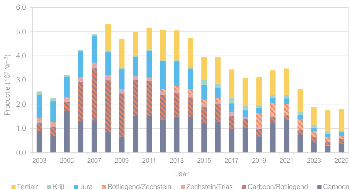
Figuur 3.4 Gasproductie op zee, per reservoir (exclusief Rotliegend en Trias reservoirs).
