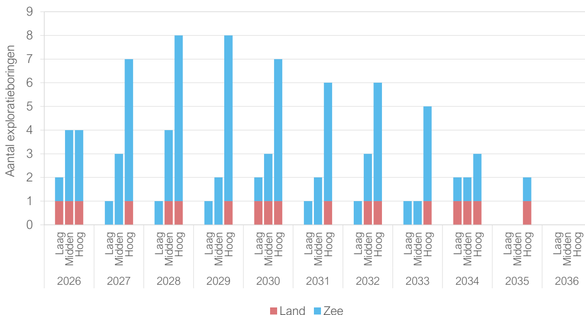
Figuur 1.4 Grafiek behorend bij Tabel 1.6: exploratie boorinspanning per scenario vanaf 2026.
