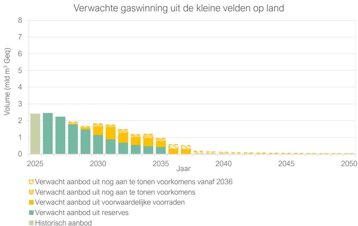
Figuur 1.5 Gerealiseerd (2025) en verwachte (2026 – 2050) winning van aardgas uit de kleine velden op land. De waarden onderliggend aan dit profiel worden in Excel overzicht tabbladen B, C en F gegeven. NB; in dit figuur is alleen het Midden scenario is weergegeven.
