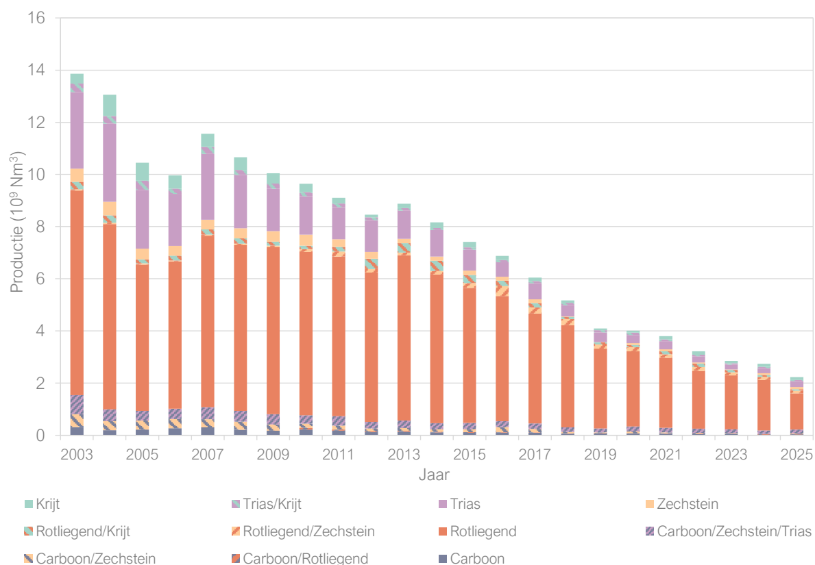
Figuur 3.1 Gasproductie op land, per reservoir (exclusief gasveld Groningen).
