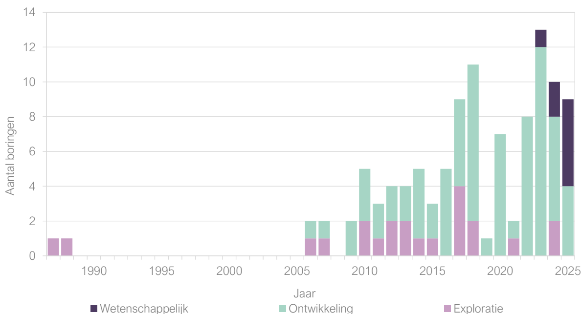
Figuur 11.4 Verloop van aardwarmteboringen op land vanaf 1987.
