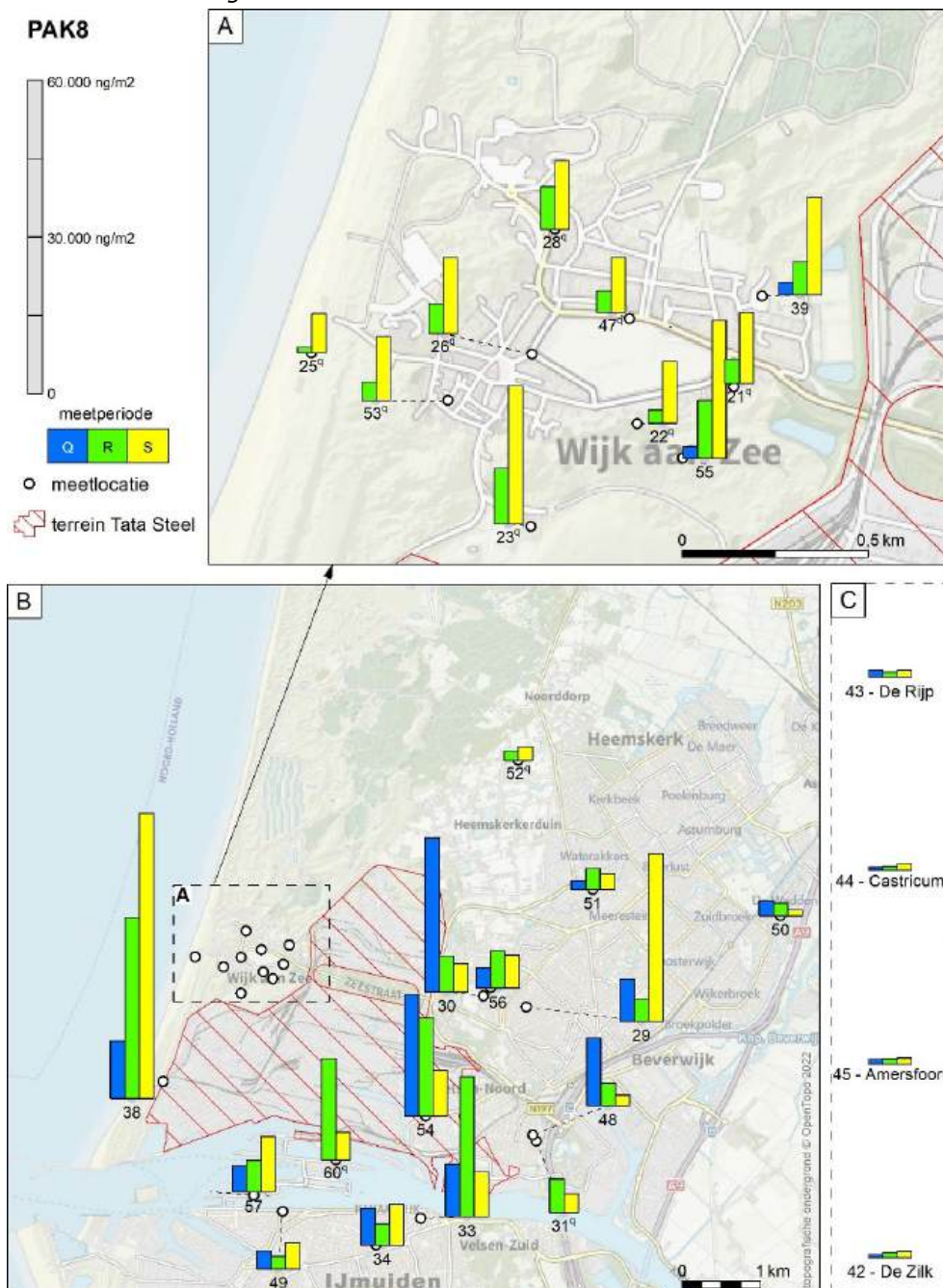
Figuur 7 Depositie van EFSA PAK8, uitgedrukt in ng/m 2 , op de locaties in de IJmond en op de vier achtergrondlocaties tijdens de drie meetperioden. Een q betekent dat op deze locatie in periode Q de bak is omgevallen en dat deze waarde niet wordt getoond.
