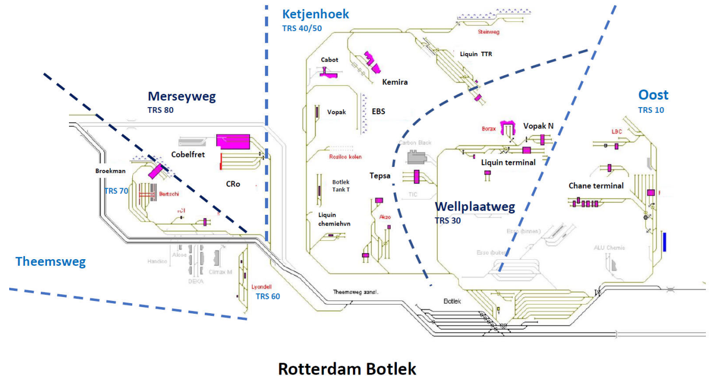
Spoorinfrastructuur in de Botlek en bijbehorende TRS gebieden (gebaseerd op Sporenplan.nl).
