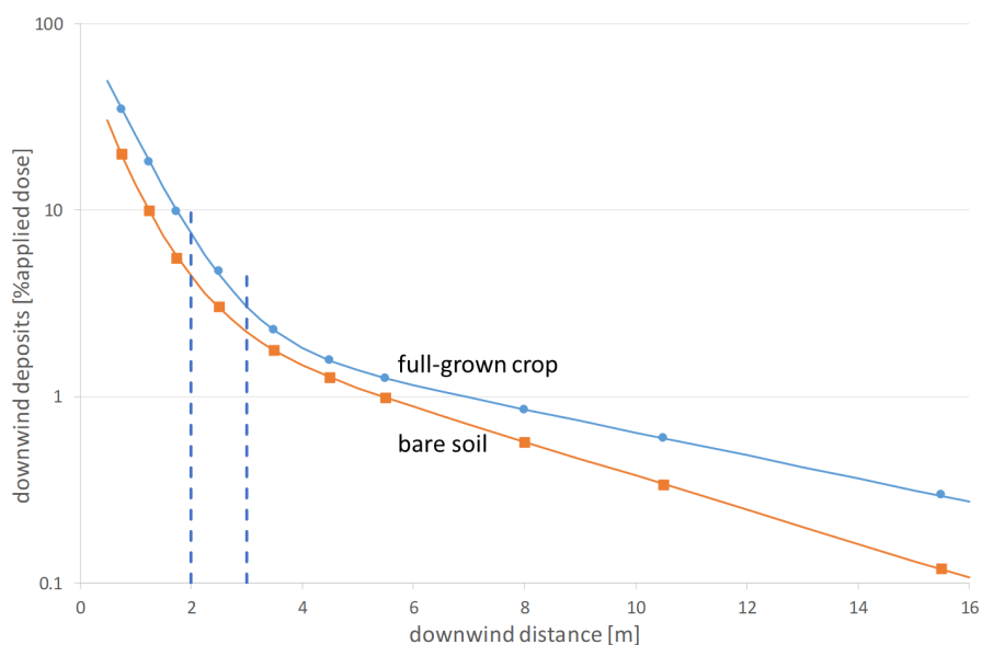
Figuur B1.2 Voorbeeld van curves van driftdepositie als functie van de afstand buiten de perceelrand, zoals gebruikt in de WUR Drift Calculator (Holterman & van de Zande, 2021). De blauwe curve geeft de driftdepositie voor een vol gewas (aardappel, 50 cm hoog); de oranje curve de driftdepositie bij een bespuiting op kale grond; beide bij een windsnelheid van ca. 3 m/s (op 2 m hoogte gemeten). De stippellijnen geven de globale ligging van een standaardslot aan (2-3 m vanaf het gewas), voor de bepaling van driftdepositie op oppervlaktewater zoals in de toelating van GBM wordt gebruikt.
