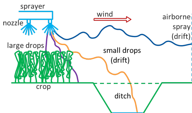
Figuur B1.1 Schematische weergave van druppelbanen in het IDEFICS driftmodel. Wegwaaiende druppels (druppeldrift) kunnen neerkomen op de grond naast het perceel (driftdepositie) of langere tijd in de lucht blijven zweven (drift naar de lucht). In het laatste geval wordt hun verdeling op een zekere afstand in het verticale vlak bepaald (rechts in de figuur).
