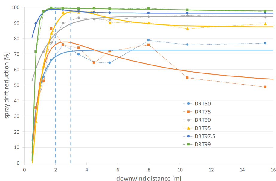
Figuur B1.5. Driftreductiecurves voor vol gewas bij neerwaartse bespuiting, als functie van de afstand. Voor driftreductieklassen DRT50 t/m DRT99. De evaluatiestrook voor de DRT-klassen ligt op afstand 2-3 m, aangegeven door de gestreepte lijnen. Dit komt overeen met de positie van het wateroppervlak van de standaardsloot bij akkerbouwmatige teelten (Holterman & van de Zande, 2021).
