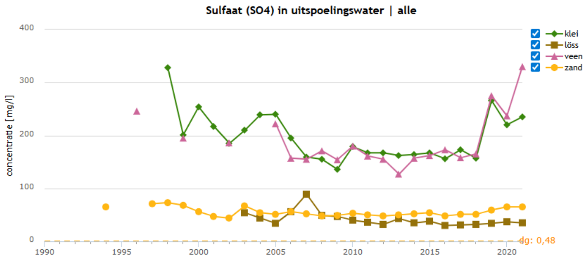
Figuur 3 Trend in de sulfaatconcentratie in uitspoelingswater op landbouwgronden uit het monitoringsnetwerk LMM ( Imm.rivm.nl ). Concentratie sulfaat in \text{mg SO}_4 \text{ L}^{-1} per grondsoort, gemiddeld over alle bedrijfstypen.
