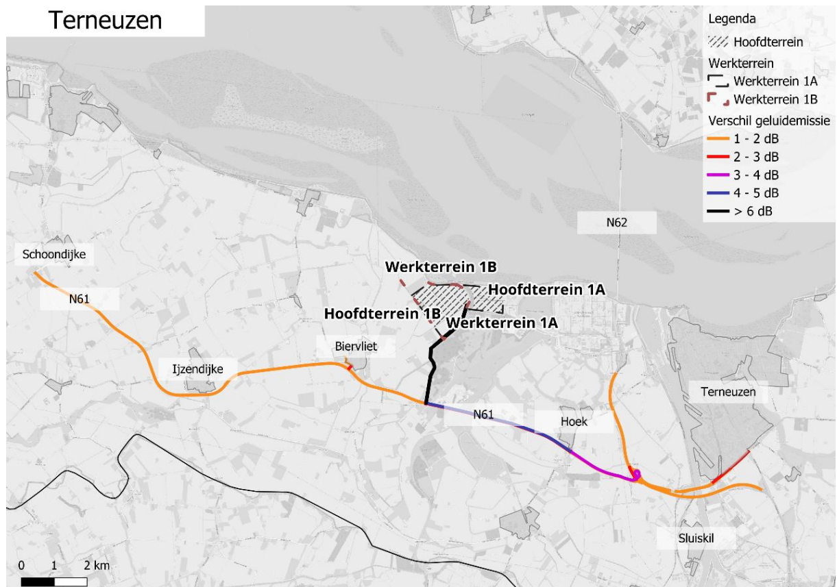
Figuur 8-6 Toename verkeerslawaaai bij Terneuzen in de bouwphase ten opzichte van de referentiesituatie (zonder verkeersmaatregelen)
