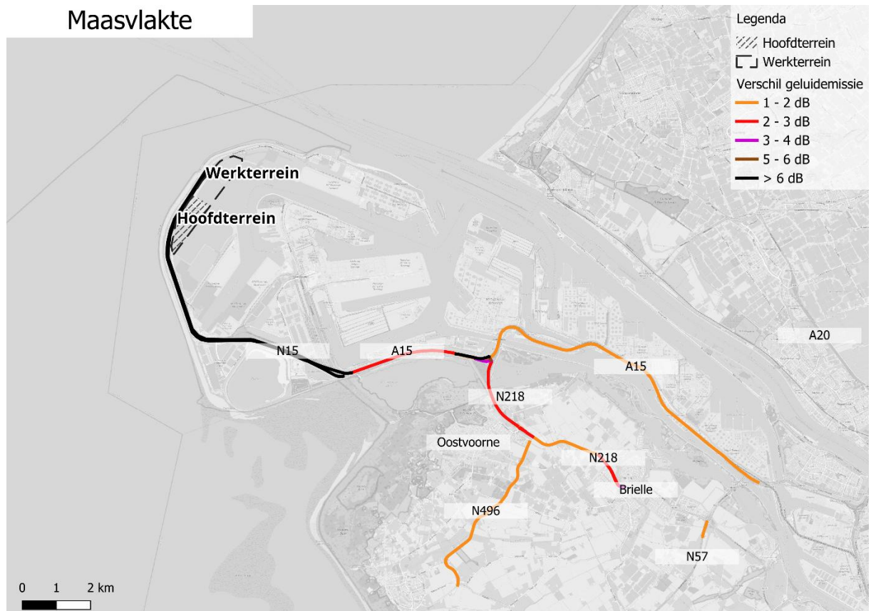
Figuur 8-3 Toename verkeerslawaaï bij Maasvlakte II in de bouwfase ten opzichte van de referentiesituatie (zonder verkeersmaatregelen)
