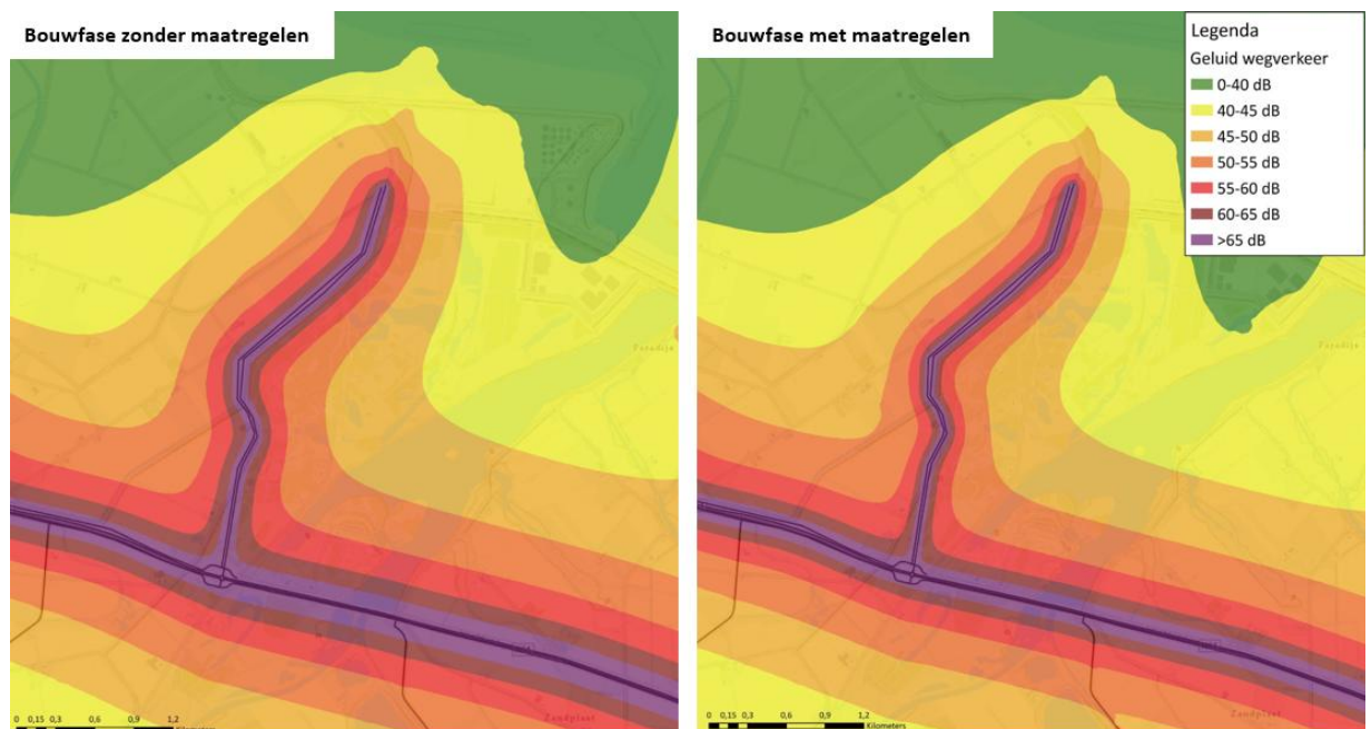
Figuur 20-3 Geluidemissie van voertuigen op de nieuwe ontsluitingsweg van het werkterrein naar de N61. Bouwfase zonder (links) en met (rechts) mobiliteitsmaatregelen
