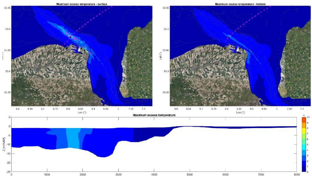
Figuur 15-5 Berekende stijging watertemperatuur door de lozing van koelwater bij Eemshaven 1A en 1B (bron: Deltares)
