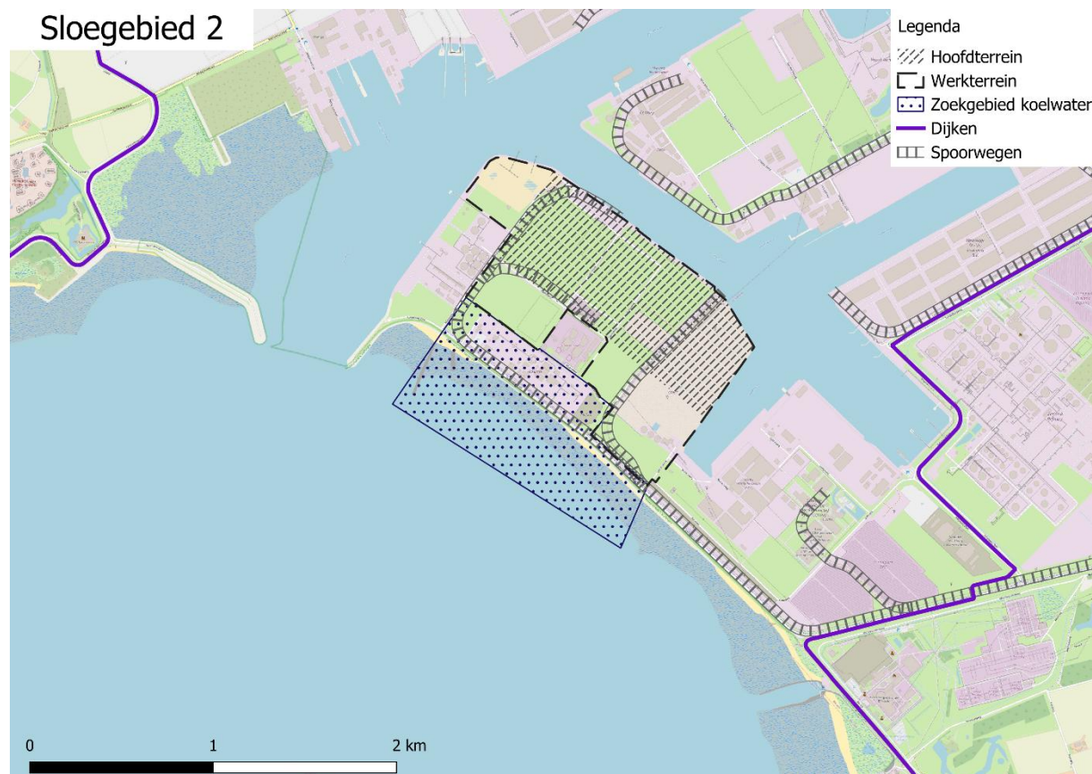
Figuur 4-23 Alternatief Sloegebied 2
