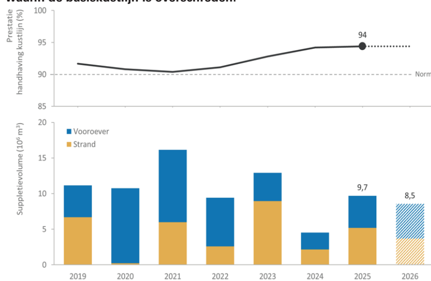
Figuur 4 Jaarlijkse hoeveelheden zandsuppleties en percentages raaien waarin de basiskustlijn is overschreden.
