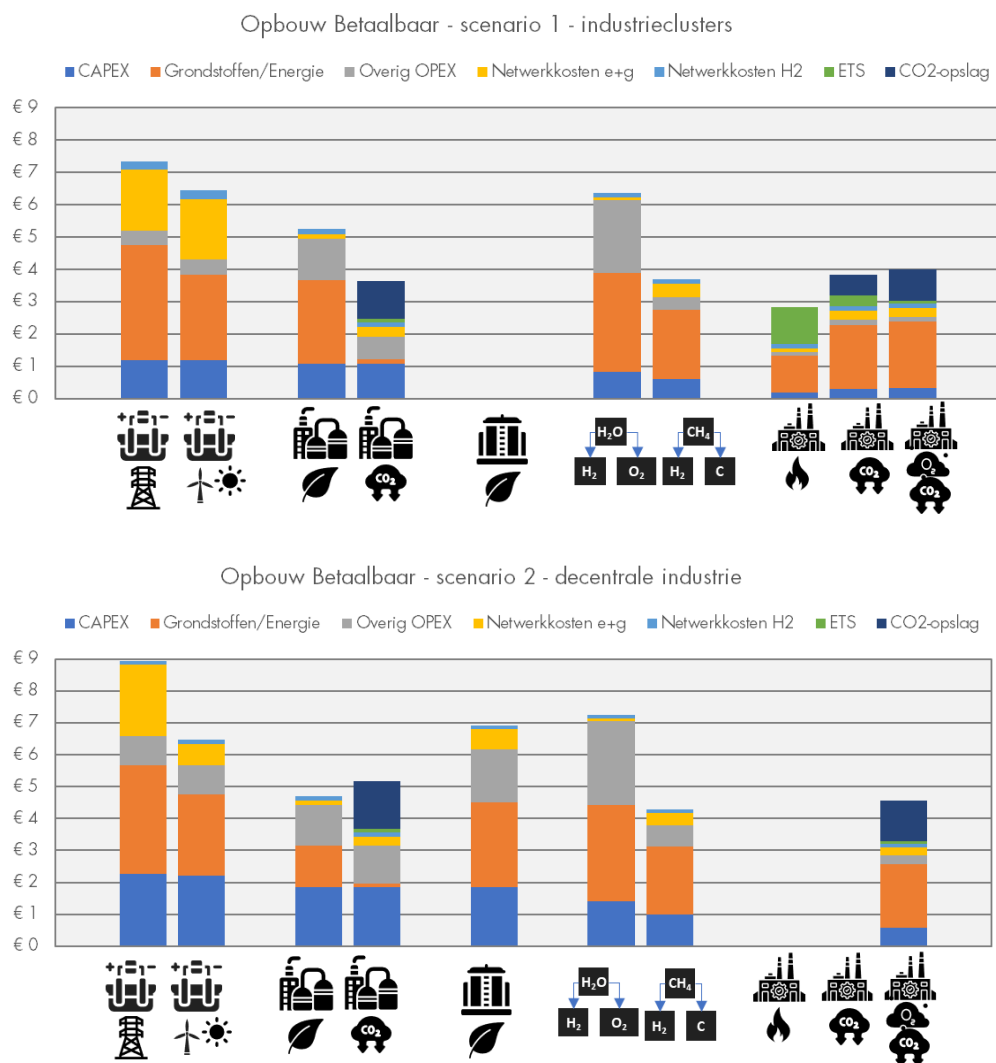
Figuur 36: Opbouw kosten per waterstofproductietechniek
