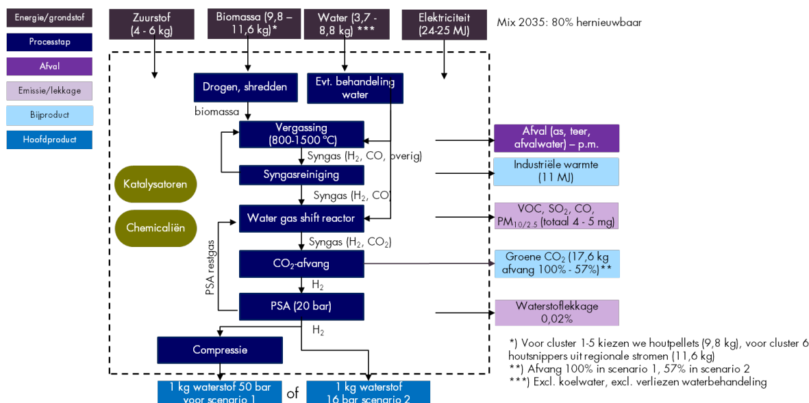
Figuur 29: Processchema vergassing van houtresten
