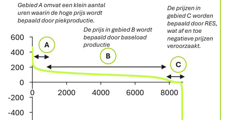
Figuur 17: Illustratieve prijsduurcurve [EUR/MWh] voor NL¹.
