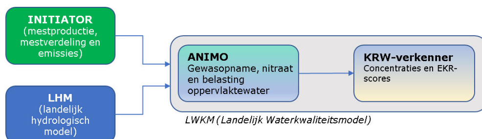
Figuur B3.1 Schema van gekoppelde modellen in het Landelijk Waterkwaliteitsmodel
