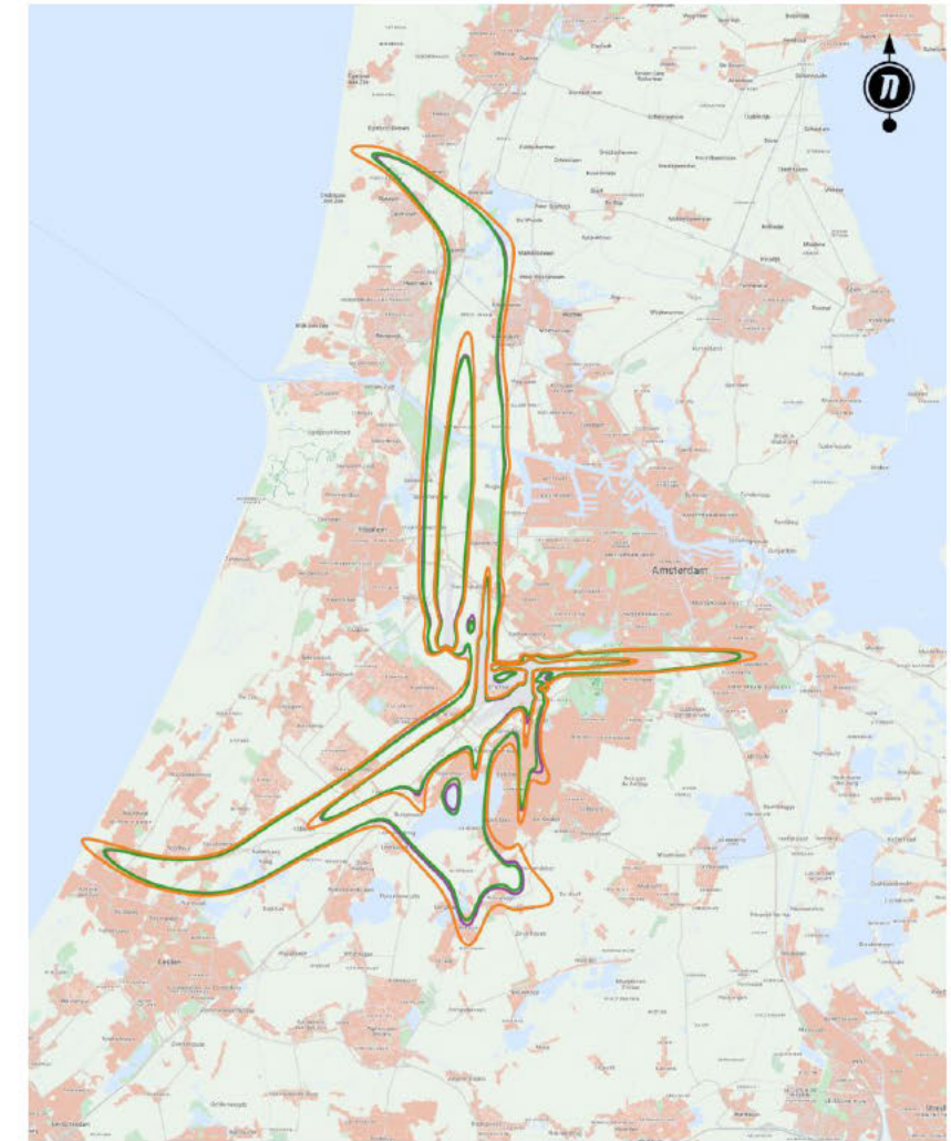
Lnight — VA2-2024 (Lnight) — VA2-2030 (Lnight) — VA2-2024 + 6 jaar autonome vlootontwikkeling (Lnight)
