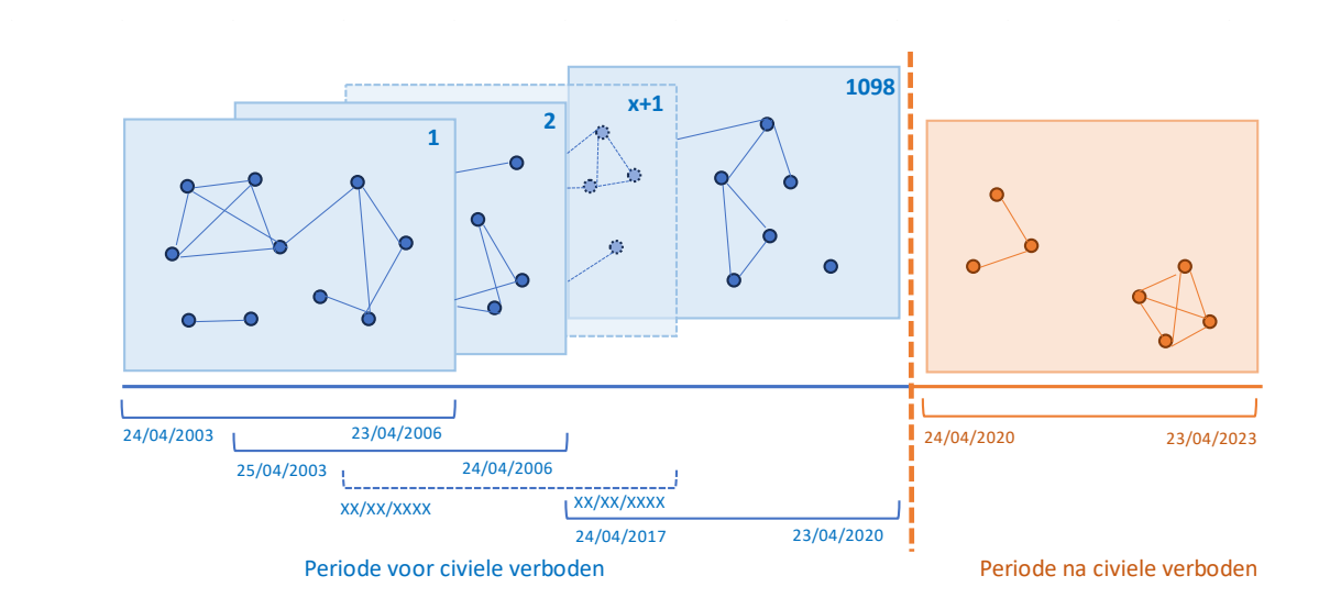
Figuur 18. Schematische weergave van de gehanteerde analyse strategie
