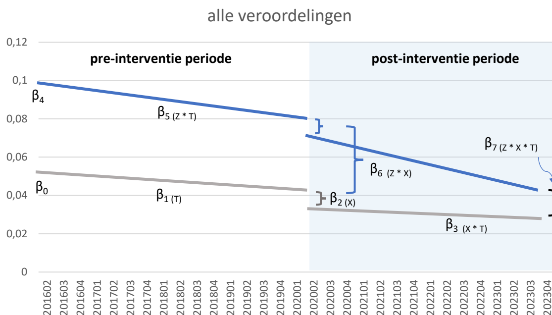
Figuur 14. Standaard regressiemodel met vergelijkgroep
