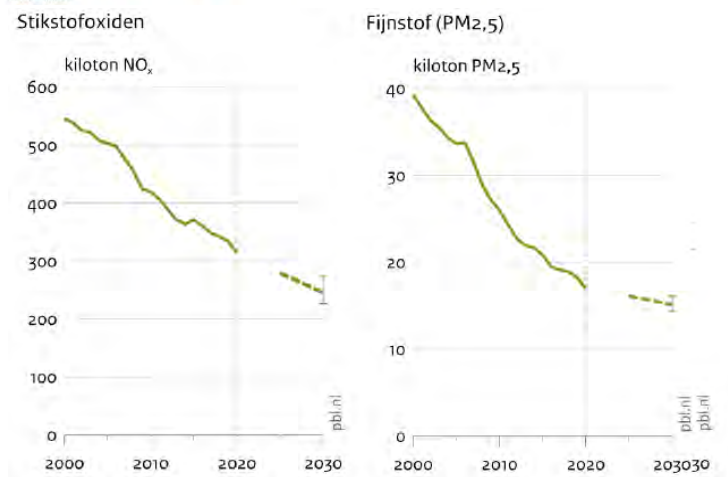
Figuur 1.12 Ontwikkeling emissie NOx en PM 2,5 tot 2030 (PBL, 2023)
