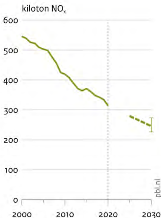
Figuur 5.25: Prognose emissie van luchtverontreinigende stoffen (Bron: PBL, 2023)
