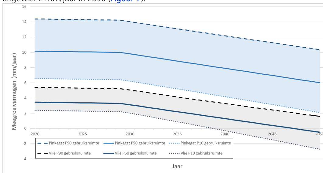
Figuur 7: Gebruiksruimteverdeling (P90-P50-P10) zonder belasting. De verdeling toont de doorwerking van de invoerverdeling van de relatieve zeespiegelstijging (uit Tabel 1 en Figuur 5 , inclusief de (kunstmatige) knik bij de overgang van het beleids- naar het richtscenario. In lichtblauw de verdeling (P10-P90) van de komberging Pinkegat en lichtgrijs (P10-P90) van de komberging Vlie.
