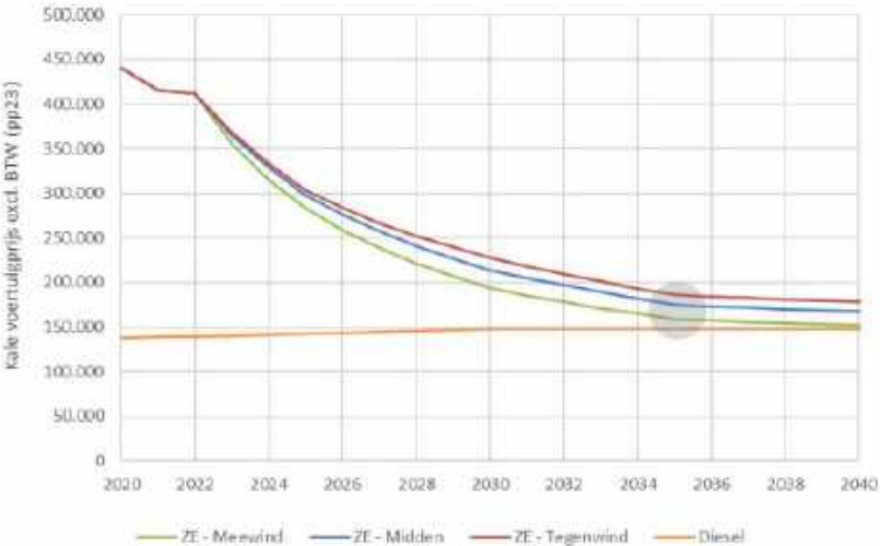
Prognose gemiddelde aanschafprijs vrachtoetuigen tussen 2020 en 2040. Bron Achtergrondrapport wagenparkanalyses bestel- en vrachtoeto's. (2024). PBL.
