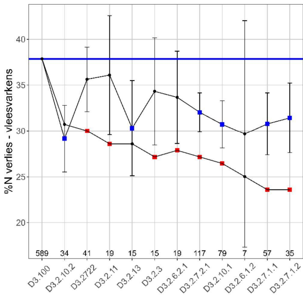
Figuur 7 Vleesvarkens: effect van staltypen op het N-verlies als percentage van de totale N-excretie, met op de horizontale as de Rav-codes van de staltypen en bijbehorend aantal bedrijven. De punten op de zwarte lijn geven per staltype de hoogte van het waargenomen N-verlies weer, en de bijbehorende verticale lijn de bandbreedte van het 99%-betrouwbaarheidsinterval. De blauwe lijn geeft het niveau van referentiestal D3.100, en de punten op de onderste lijn het volgens de Rav-factor verwachte \text{NH}_3\text{-N} verlies per staltype t.o.v. de referentiestal. Staltypen met significant hogere verliezen dan verwacht volgens de Rav-factor zijn gemarkeerd met rode vierkanten op de verwachtingslijn. Significant afwijkende (lagere) verliezen dan de referentiestal zijn gemarkeerd met blauwe vierkanten op de lijn met de waargenomen verliezen.
