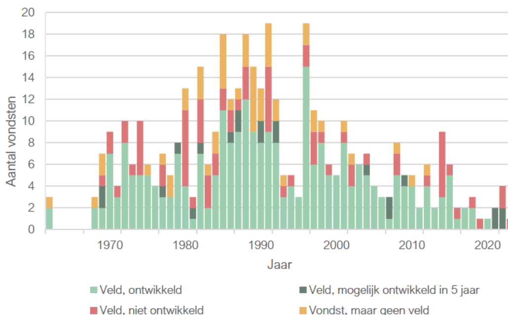
Figuur 7: Vondsten van koolwaterstoffen in Nederland offshore per jaar en onderverdeeld in ontwikkeld veld, (nog) niet ontwikkeld veld of niet geclassificeerd als veld.
