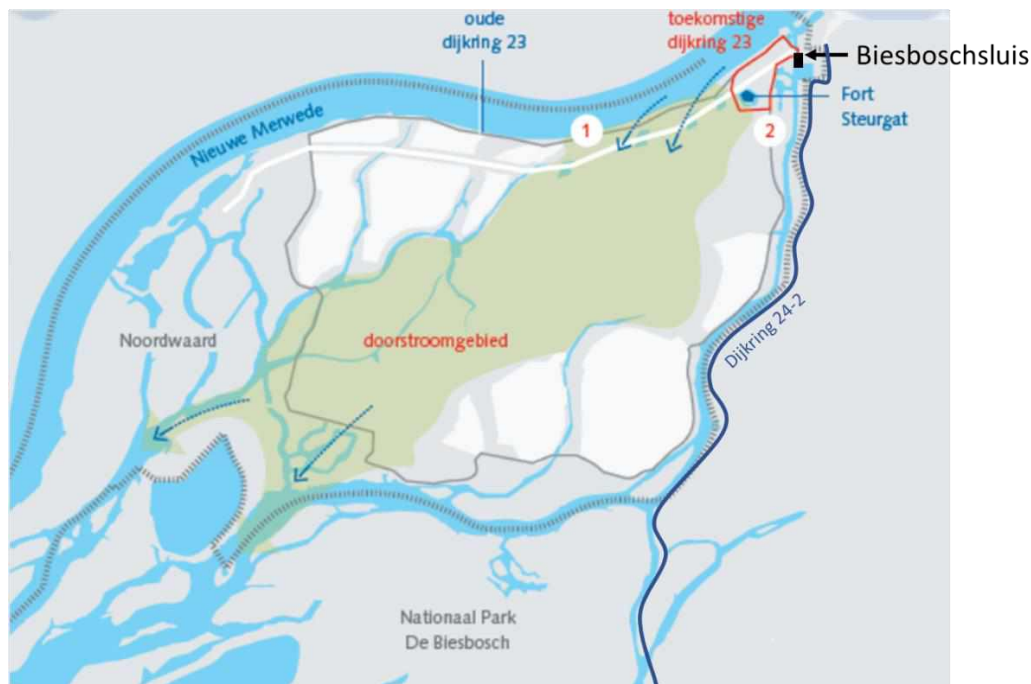
Figuur 3-2 Ruimte voor de Rivier-maatregel dijkkring 23.
