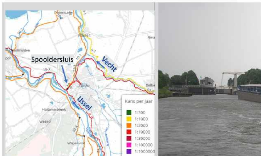
Figuur 2-1 Ligging en foto van de Spooldersluis.
