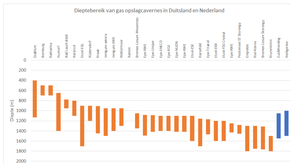
Figuur 9.4 Overzicht van het dieptebereik, waarbinnen bestaande opslagcavernes in Duitsland (oranje) en Nederland (blauw) zijn aangelegd. Bronnen: i) https://www.lbeg.niedersachsen.de/download/177852/Untertage-Gasspeicherung_in_Deutschland_Stand_1.1.2021_.pdf en ii) Opslagplannen Zuidwending en Heiligerlee ( www.nlog.nl ).
