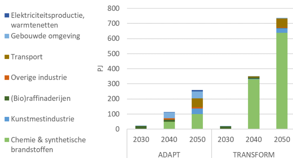
Figuur 4.1 Waterstofverbruik in 2030 tot 2050 volgens ADAPT- en TRANSFORM-scenario's. De grafiek geeft de waterstof weer, die extern kan worden geleverd en is exclusief de waterstof, die ontstaat en wordt gebruikt binnen chemische processen.
