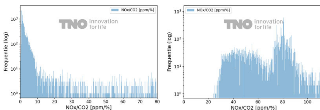
Figuur 8: Histogram \text{NO}_x/\text{CO}_2 ratio van machine met SCR-katalysator (links) en machine zonder SCR-katalysator (rechts), y-as is logaritmisch.
