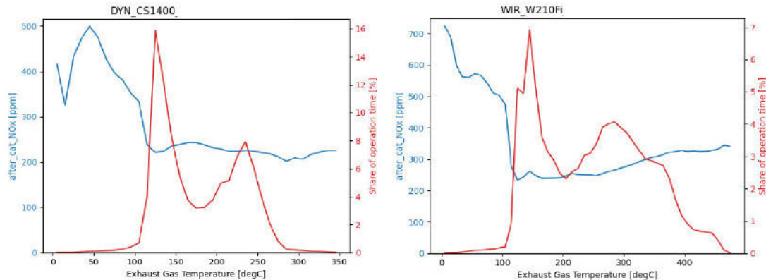
Figuur 7: \text{NO}_x -concentratie (blauwe lijn) en tijdsaandeel (rode lijn) als functie van de uitlaatgastemperatuur voor vier Stage V machines zonder een SCR-katalysator.
