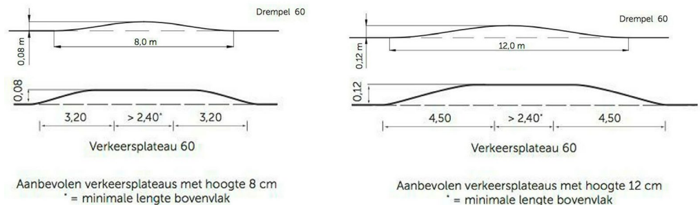
Afbeelding 5.8. Verticale snelheidsremmers op erftoegangswegen buiten de bebouwde kom (CROW, 2021)
