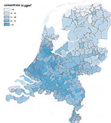
NO 2 , 2017
