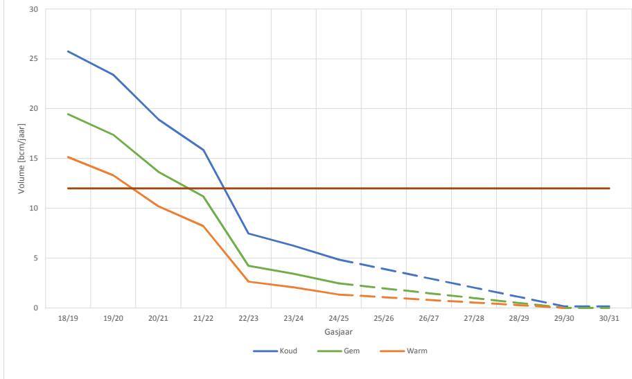
Figuur 2: Groningen volume bij ombouw 53 grootverbruikers en plaatsing stikstofinstallatie
