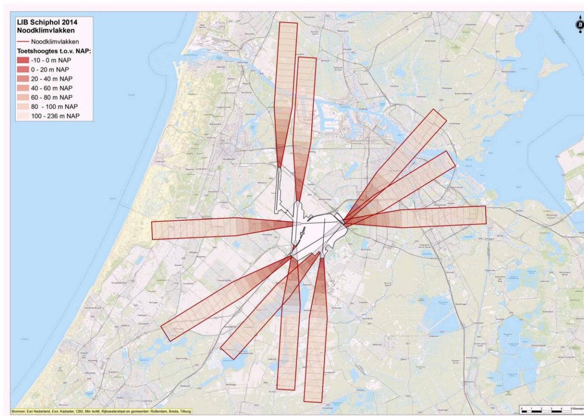
Figuur 1. Noodklimvlakken
