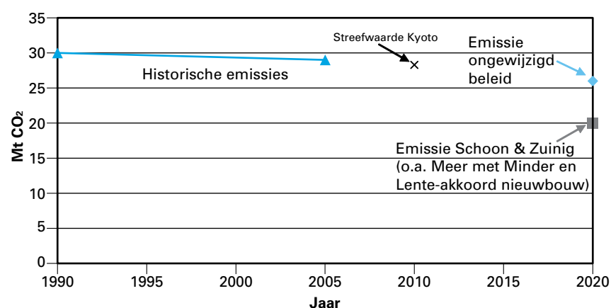
Grafiek 2.2. Ontwikkeling CO 2 emissies gebouwde omgeving
